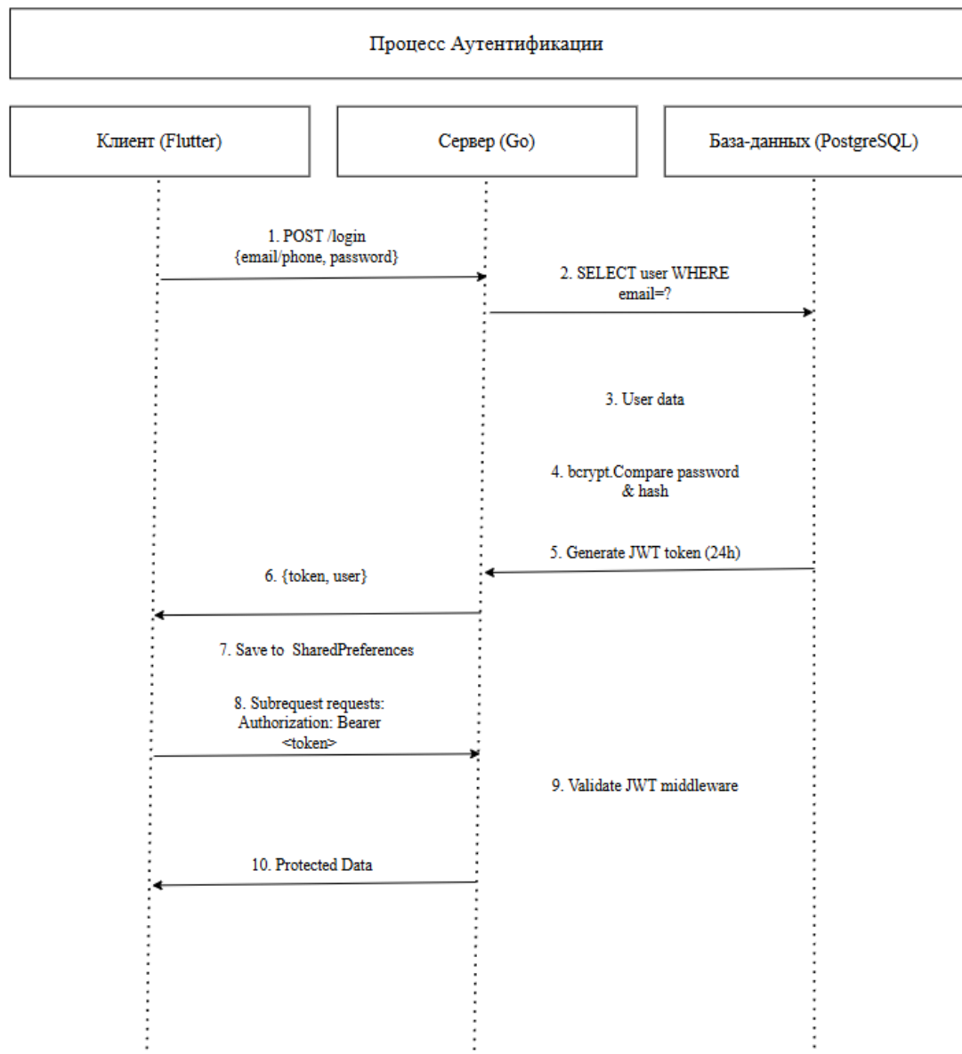
Рисунок 3.5 – Процесс аутентификации пользователя
